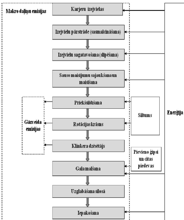
1. attēls. Cementa ražošanas procesa diagramma, kas ietver enerģijas un siltuma patēriņa nepieciešamību noteiktiem procesa etapiem, kā arī makrodaļiņu un gāzveida emisijas
