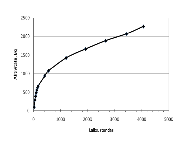
1. attēls. ^{137}\text{Cs} izdalīšanās līkne stacionārajā režīmā. Temperatūra 20 \pm 1^\circ\text{C}
