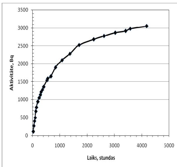
2. attēls. ^{137}\text{Cs} izdalīšanās līkne plūsmas režīmā. Temperatūra 20 \pm 1^\circ\text{C}
