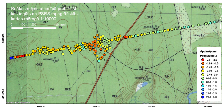
2. attēls. Reālais reljefs attiecībā pret digitālo reljefa modeli, kas iegūts no PSRS topogrāfiskās kartes mērogā 1:10 000 reljefa slāņā
