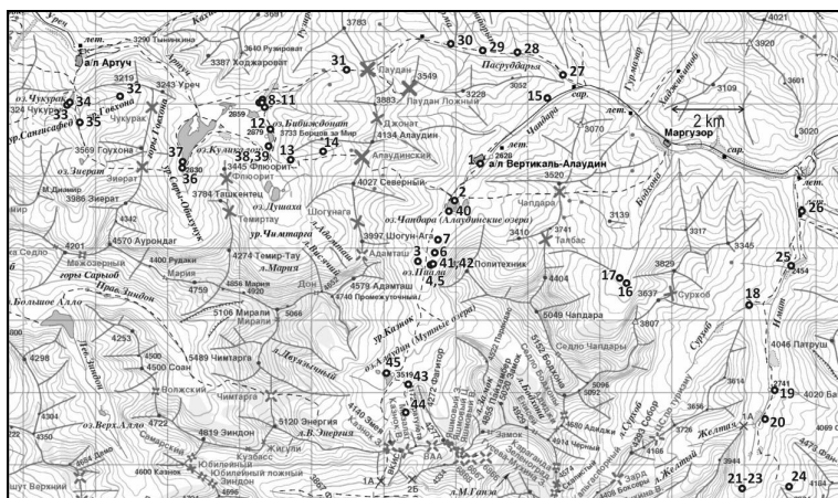
1. attēls. Virszemes un pazemes ūdeņu fizikāli ķīmisko parametru novērojumu punkti Fanu kalnos
