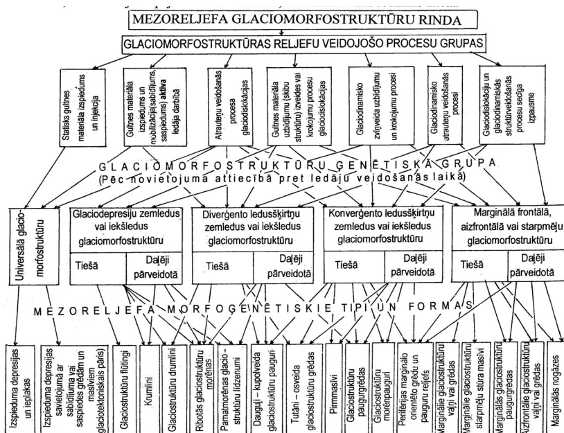
1. attēls. Glaciomorfostuktūru mezoreljefa ģenētiskās rindas iedalījums ģenētiskajās grupās pēc reljefa formu novietojuma attiecībā pret ledāju to veidošanās laiku
