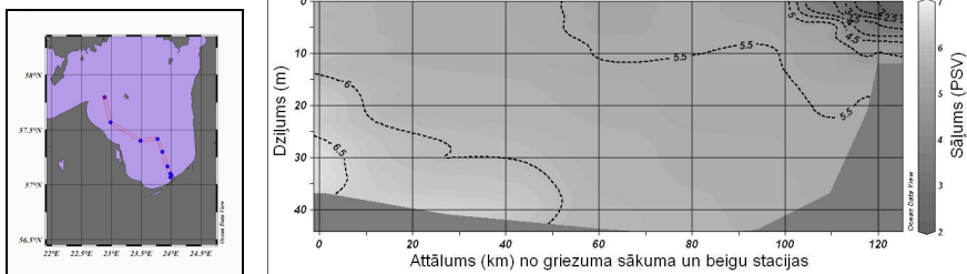
1. attēls. Ūdens sāļuma svārstības telpā (pa horizontiem) griezumā no 111. līdz 165. stacijai 2003. gada maijā
