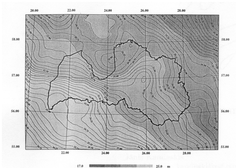
1. attēls. Latvijas ģeoīda modelis, k.i. 0,25 m
