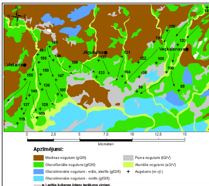
1. attēls. Vidzemes augstienes DA nogāzes kēmu terases (posms no Vietalvas līdz Aronas upes ielejai) hipsometriskā augstuma izmaiņas un ledājkušanas ūdeņu paleostraumju iespējamie virzieni
