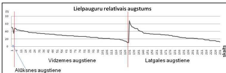
1. attēls. Plakanvirsas lielpauguru relatīvā augstuma sadalījuma grafiki dažādās Latvijas salveida akumulatīvi glaciostrukturālajās augstienēs
