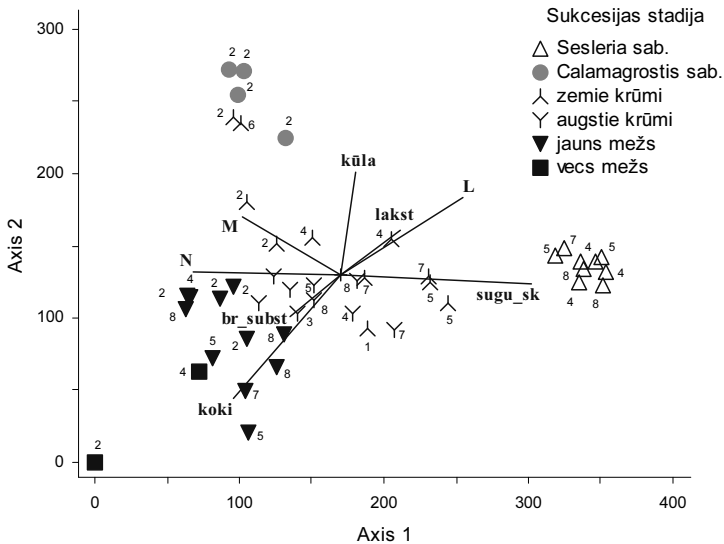
1. attēls. Veģētācijas aprakstu DCA ordinācija. 1. ass izskaidro 48% un 2. ass – 15% variācijas. Numurs (1–8) pie simboliem norāda lauces numuru, kurā apraksts veikts. Vektoru apzīmējumi: kūla – kūlas daudzums; lakst – lakstaugu stāvakopējais segums; sugu_sk – kopējais sugu skaits, br_subst – kaila zeme (%), ko nenosedz augi; koki – koku stāva segums, M, N un L – Ellenberga indikatorvērtības attiecīgi mitrumam, slāpeklim un gaismai.
