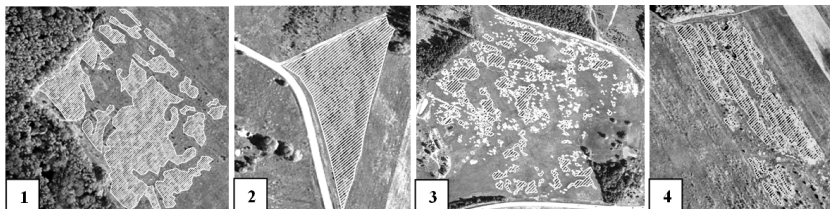
1. attēls. Ainavekoloģiskās sukcesijas attīstība neapsaimniekotajās lauksaimniecības zemēs Siguldā–Ieriķu apkārtnē: 1 – ainavekoloģiskās sukcesijas attīstība no mežmalas; 2 – vienlaidus ainavekoloģiskās sukcesijas attīstība; 3 – mozaīkveida ainavekoloģiskās sukcesijas attīstība; 4 – lineāra ainavekoloģiskās sukcesijas attīstība
