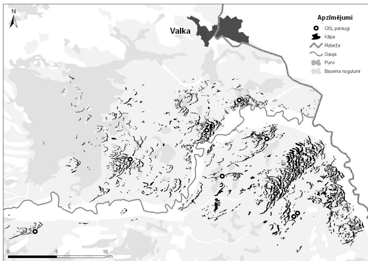
1. attēls. Iekšzemes kāpas Sēdas līdzenumā un OSL datējumu paraugu ņemšanas vietas
