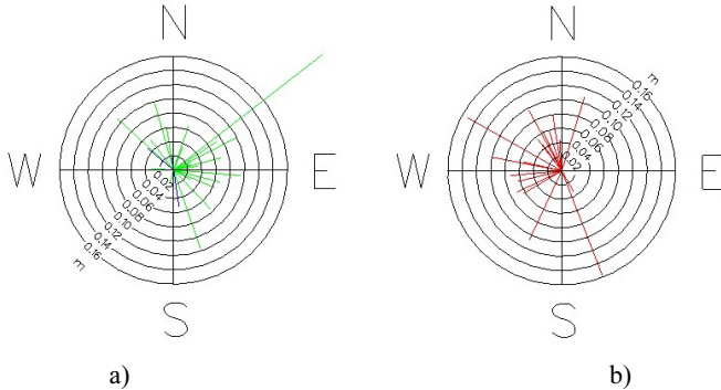
1. attēls. Poligonometrijas punktu koordinātu nobīžu vektoru rozes veida diagrammas
