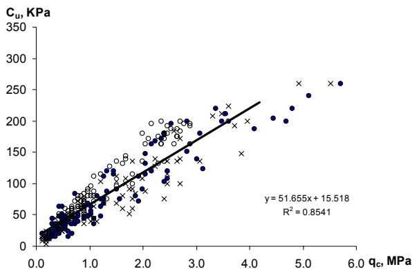
3. attēls. Konusa pieres pretestības un lāpstiņu griezes bīdes pretestības mērījumu rezultātu savstarpējās atkarības.
