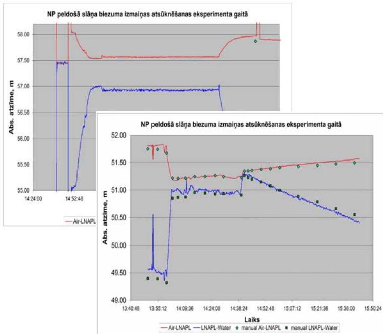
2. attēls. Eksperimentu gaitā noteiktās naftas produktu peldošā slāņa biezuma izmaiņu līknes.
