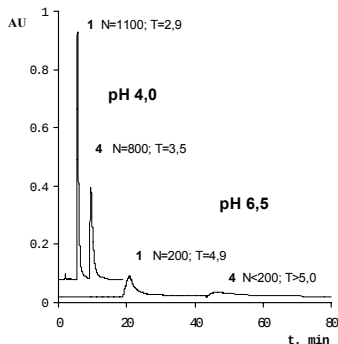
4. attēls. 1-(2-Metoksietil)-3-metilimidazoliņa hlorīda (1) un 1-benzil-3-metilimidazoliņa hlorīda (4) hromatogrammas uzņemtas 0,01 M NaH_2PO_4/CH_3OH (85:15) pie pH=4,0 un pH=6,5 .
