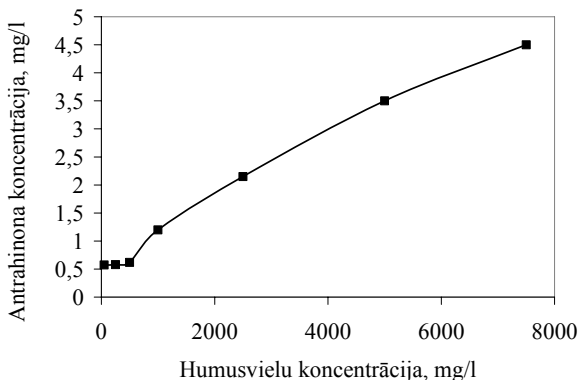
2. attēls. Humusvielu spējas šķīdināt mazšķīstošu hidrofobu organisko vielu – antrahinonu.
