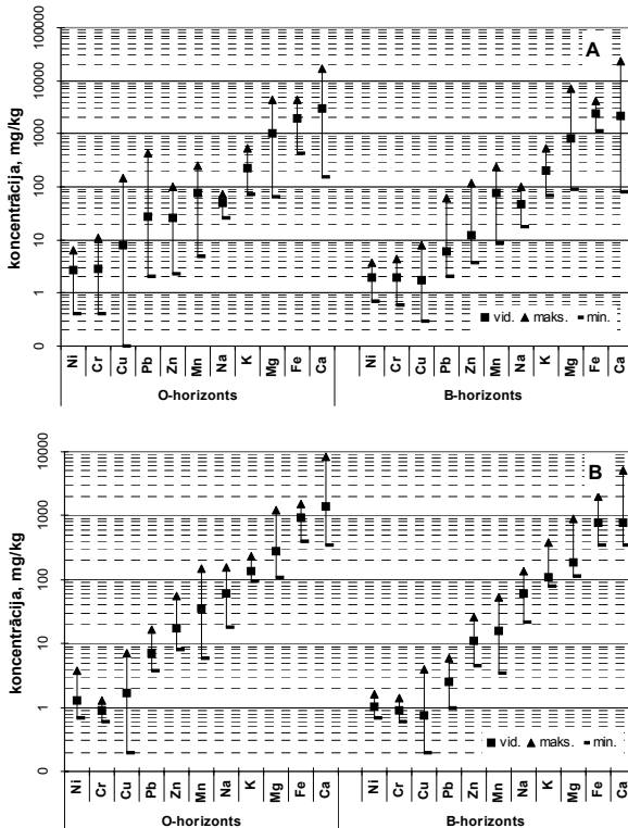
1. attēls. Makro- un mikroelementu koncentrācija Šķēdes (A) un Strautiņu (B) poligona augsnēs.
