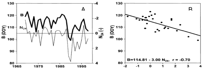
1. attēls. A. Augšanas sezonas sākuma (melnā līnija) un februāra–aprīļa NAO (N 24 ) indeksa (pelēkā līnija) trendi (1989.-1998. gads); B. Korelācija starp šiem diviem lielumiem (Chmielewski and Rotzer, 2001); DOY- dienas no gada sākuma.
