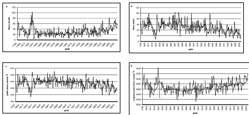
1. attēls. Temperatūras indeksu gada vērtības un 5 gadu slidošās vidējās vērtības. (a) Silto dienu skaits (b) auksto dienu skaits; (c) apkures grādu dienu summa; (d) augšanas grādu dienu summa.
