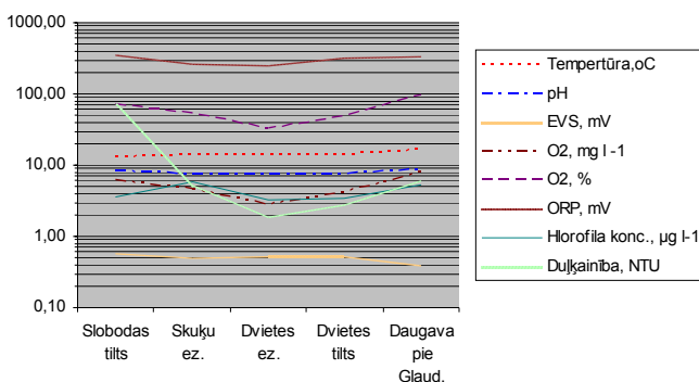
1. attēls. Fizikāli ķīmisko parametru vidējo vērtību atšķirības starp Dvietes palienes ūdens objektiem.
