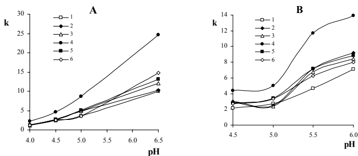
2. att. Imidazolijs atvasinājumu izdalīšanās faktora k atkarība no buferšķīduma pH vērtībām, kas iegūtas 0,01 M NaH 2 PO 4 /CH 3 OH: A - 85:15, B - 75:25 šķīdumā. Savienojumu apzīmējumus 1- 6 skat. tekstā.
