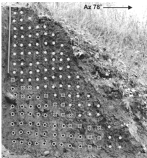
1. attēls. Konusa pieres pretestības ( q_c , MPa) rezultātu sadalījums glaciģēno grunšu atsegumā Aizputes apkārtnē. Apzīmējumi: ● – 6,0 – 2,5 MPa; × – 2,5 – 1,1 MPa; ○ – 1,1 – 0 MPa.
